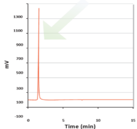
図2: rCTPのRP-HPLC溶出データ
